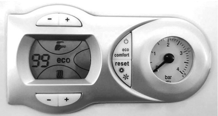
Рис. 14. Режим TEST (мощность системы отопления = 100%, индикация - 99)
