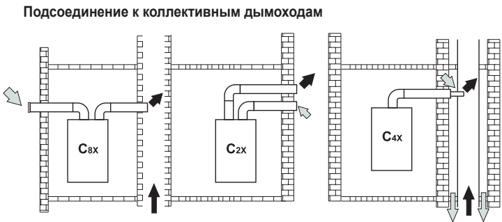
Рис. 13. Примеры подсоединения к дымоходам ⇨ – воздух; ⇩ – дымовые газы
