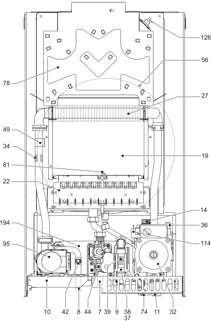
Рис. 17а. Конструкция Fortuna C32
