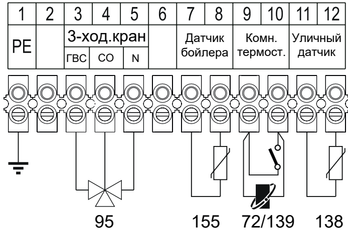
Рис. 9 Подключение внешнего опционного электрооборудования 72) Комнатный термостат 95) Трехходовой кран (подключение проводов показано условно); 138) датчик уличной температуры; 139) ПДУ с OpenTherm; 155) датчик температуры бойлера.
