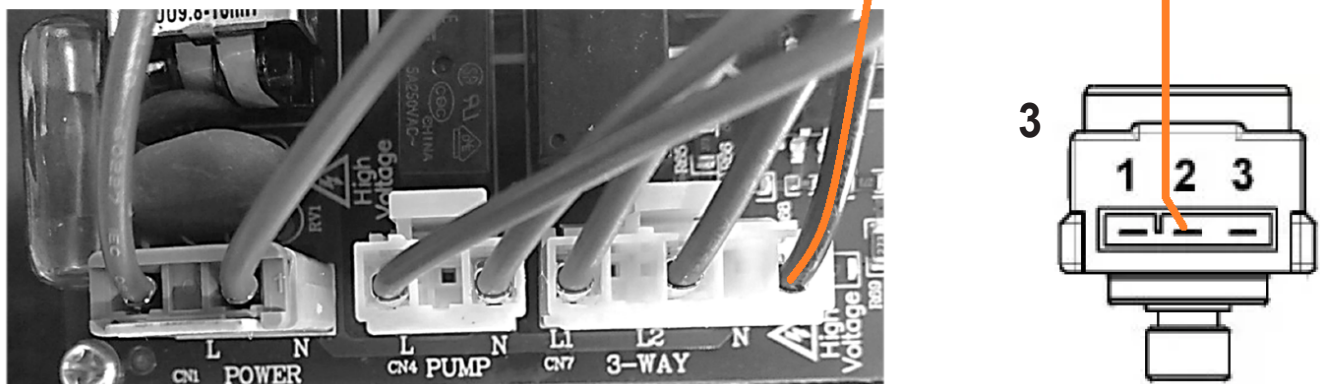
Рис. 9.1 Подключение провода "N" к электронной плате и сервоприводу
