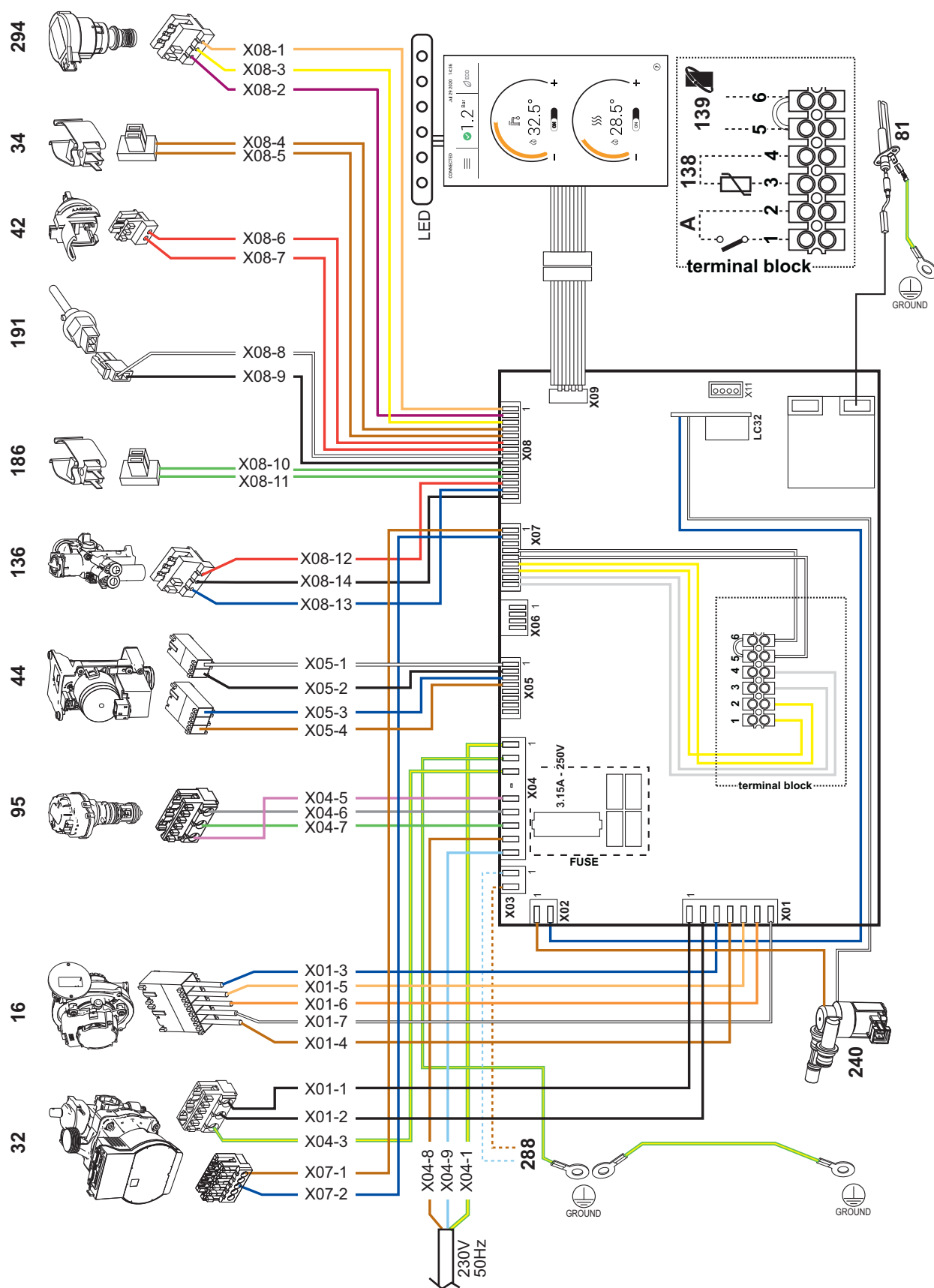
рис. 46- Электрическая схема
