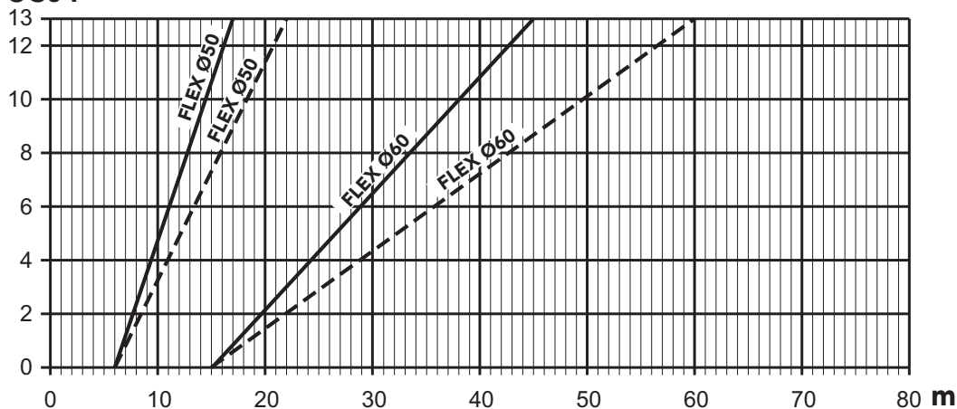
рис. 19- График выбора параметров дымохода
