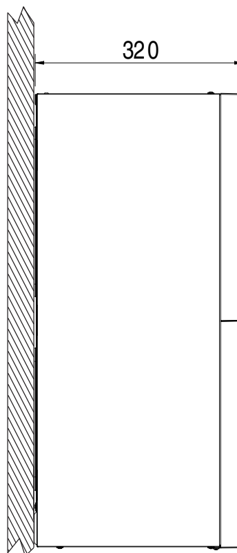
рис. 36- Вид сбоку
