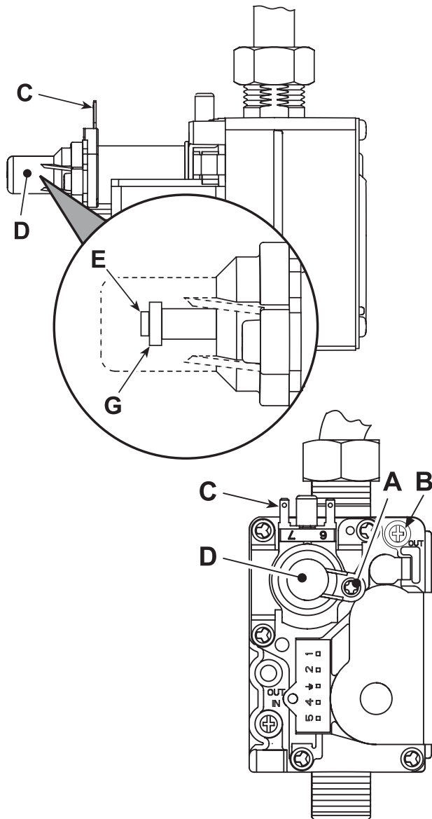
Рис. 14. Газовый клапан
