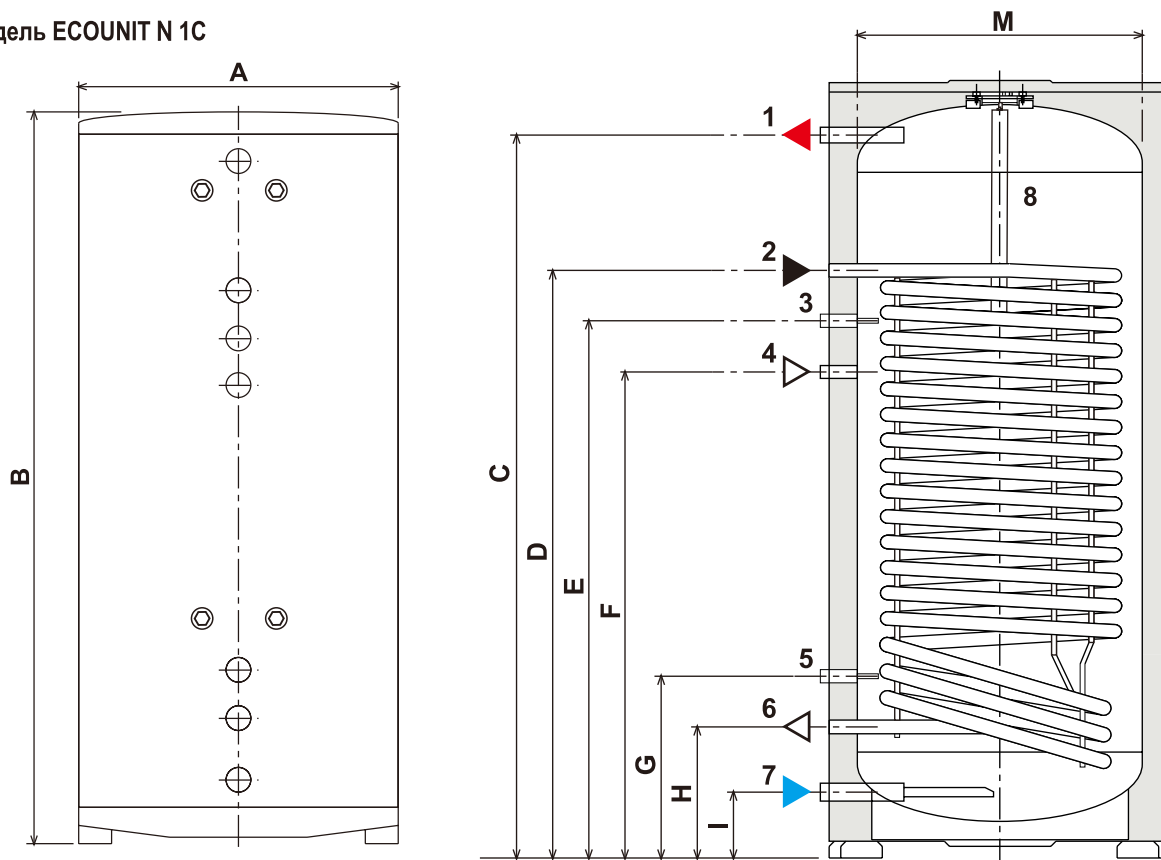
Рис. 1- ECOUNTIT N 1C
