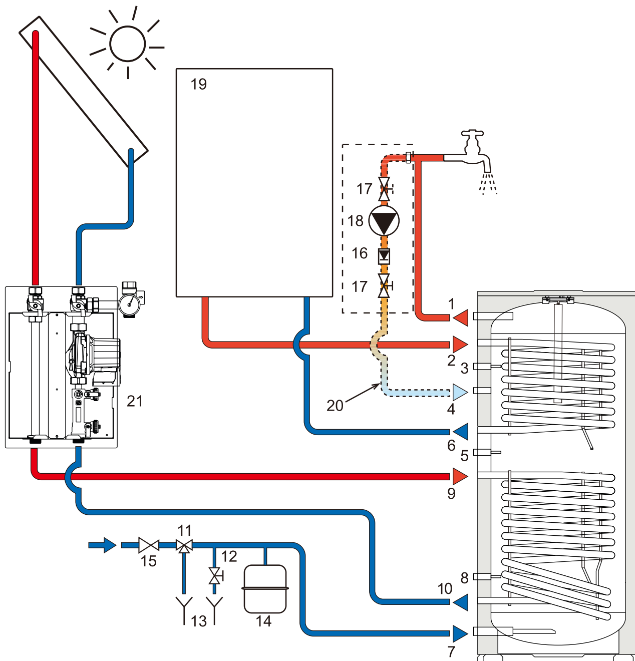
Рис. 4 – Гидравлический контур котлур ECOUNTIT N 2C
