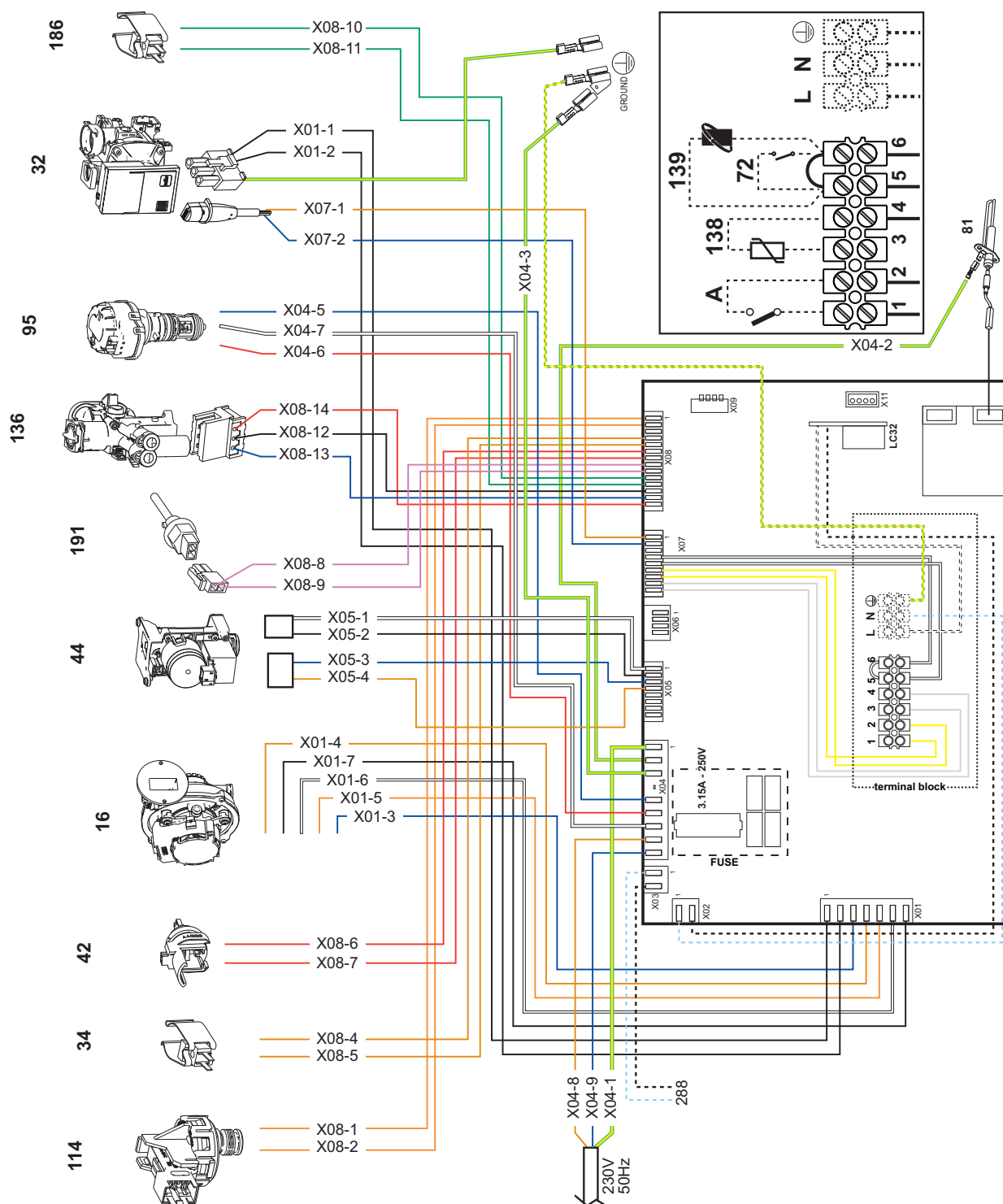
рис. 62- Электрическая схема
