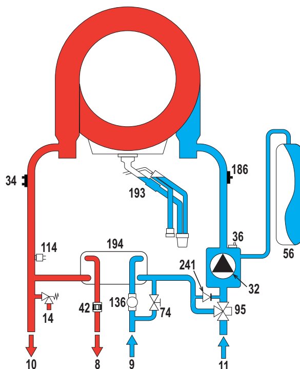
рис. 60- Гидравлический контур
