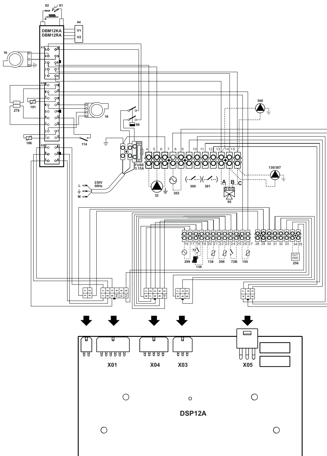
рис. 42 - Электрическая схема
