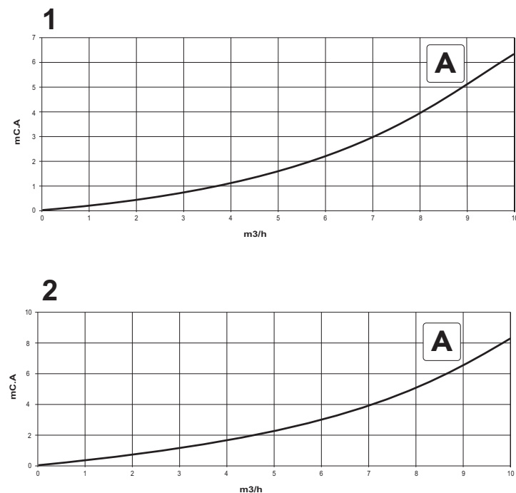
рис. 41 - Диаграммы сопротивления системы
