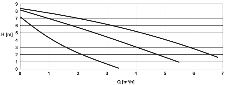
рис. 16 - Напор насоса
