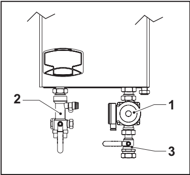
рис. 15 - Опционные комплекты
