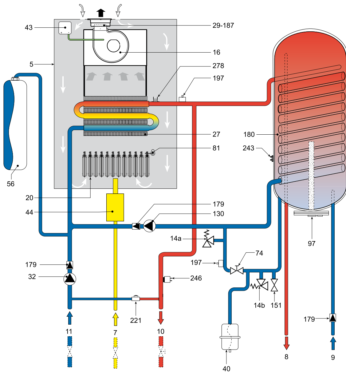
рис. 32 - Гидравлический контур
