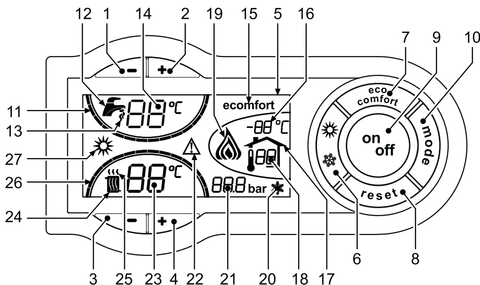
рис. 1 - Пульт управления
