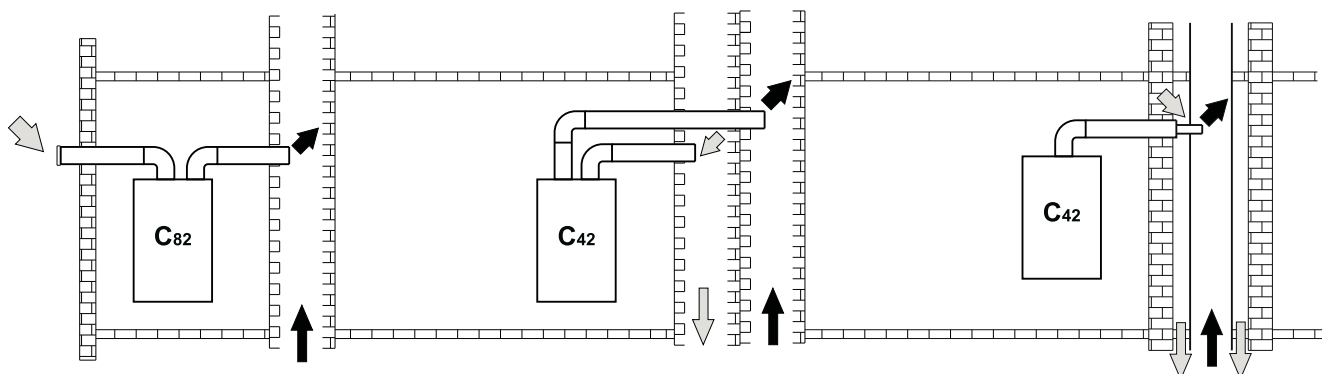
рис. 25 - Примеры подключения к дымоходам ( -воздух / - дымовые газы)
