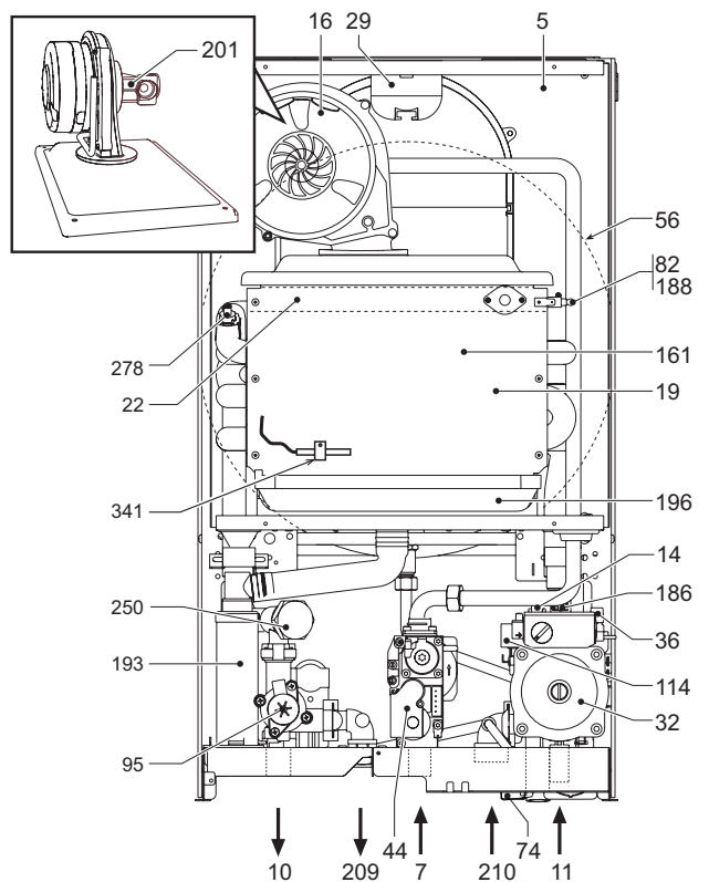
рис. 19 - Общий вид ECONCEPT TECH 25 A
