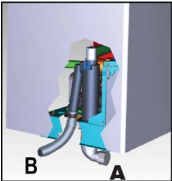
рис. 16 - Подсоединение трубы для слива конденсата
