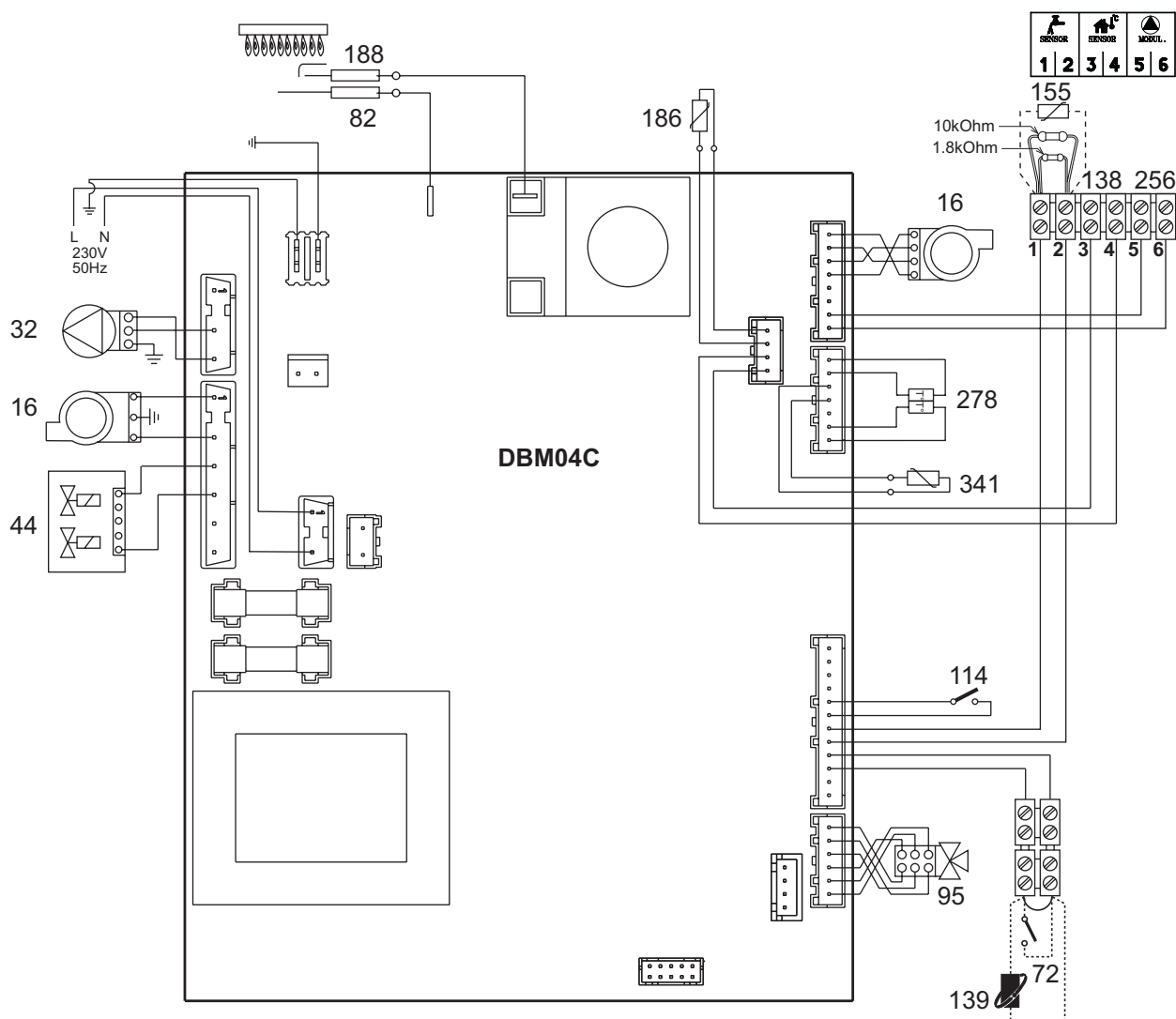
рис. 23 - Электрическая схема
