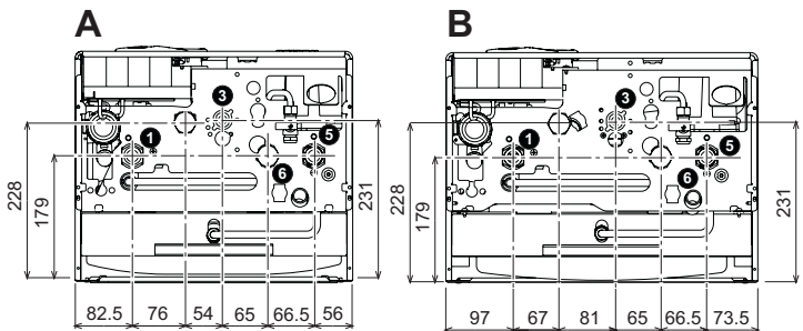
рис. 8 - Гидравлические присоединения
