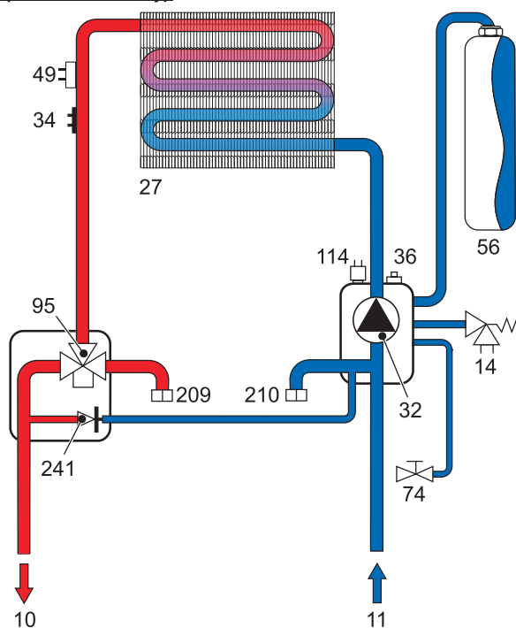
рис. 17 - Отопительный контур
