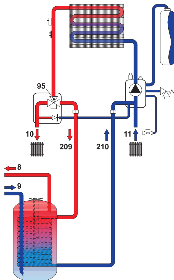
рис. 18 - Схема подключения внешнего бойлера
