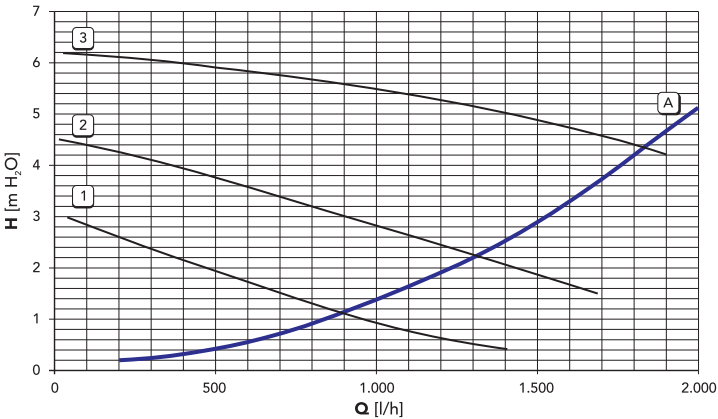
Потери напора циркуляционных насосов
