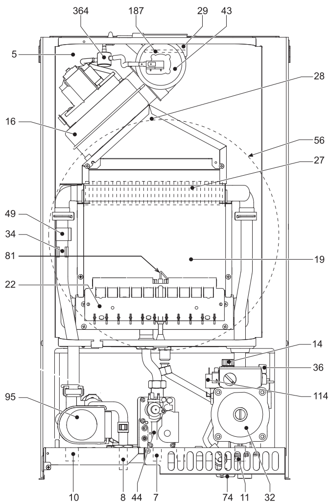
рис. 16 - Общий вид
