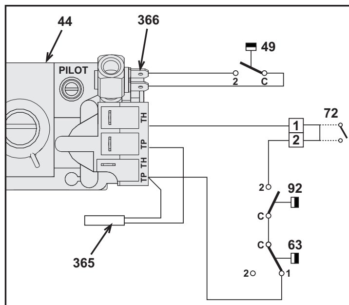
рис. 14 - Электрическая схема
