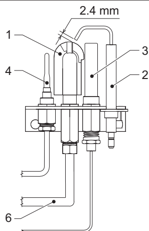
рис. 8 - Пилотная горелка
