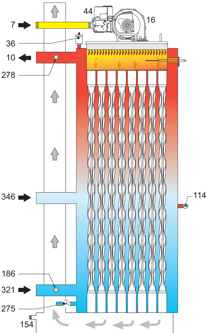
рис. 84 - Гидравлический контур
