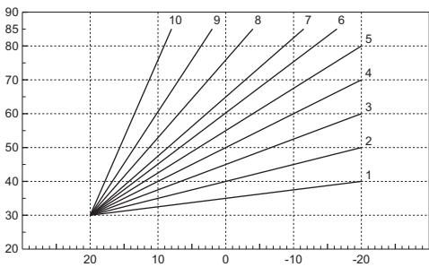
рис. 28 - Кривые погодозависимого регулирования
