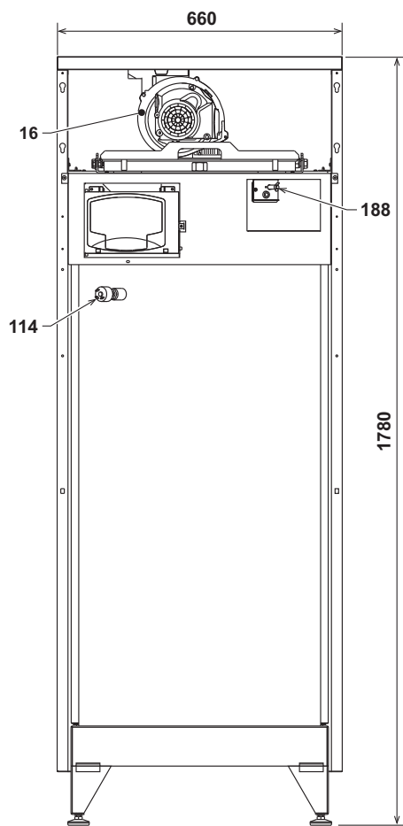
рис. 72 - Вид спереди модели B 125
