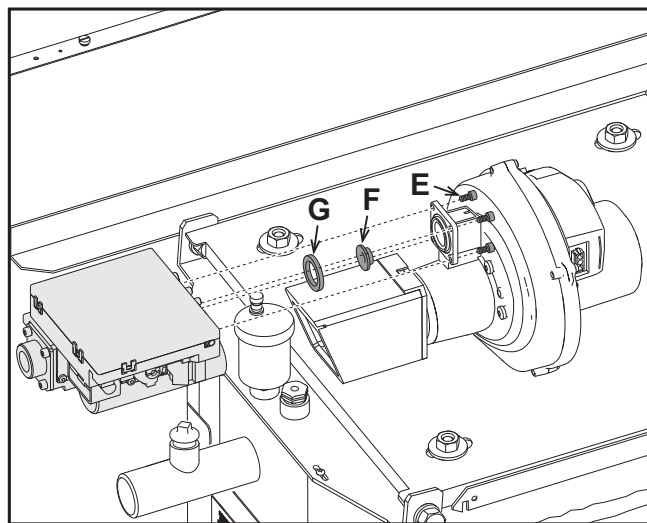
рис. 60 - Модель QUADRIFOGLIO B 125
