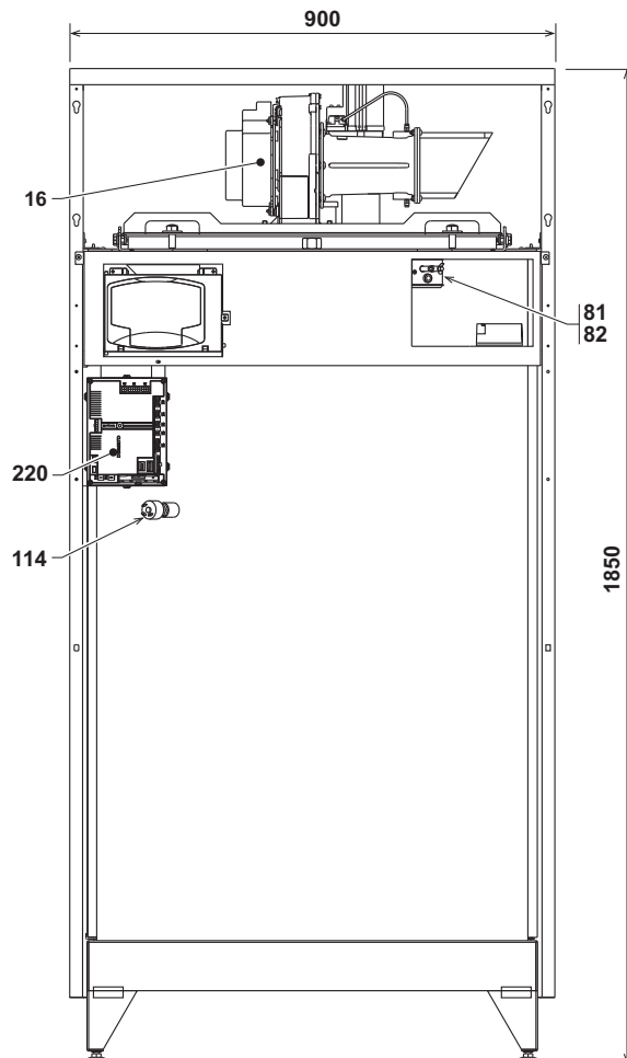
рис. 74 - Вид спереди модели B 320
