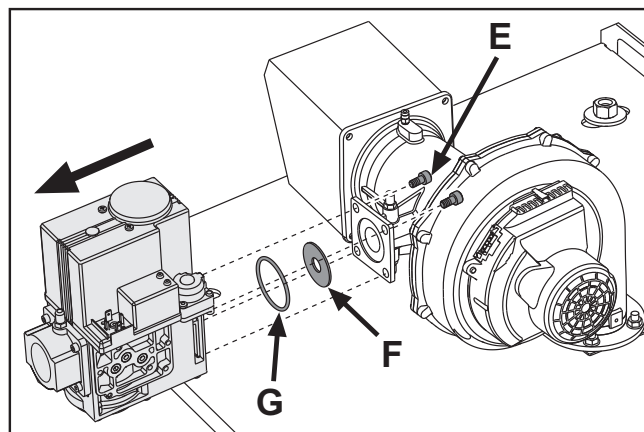
рис. 61 - Модель QUADRIFOGLIO B 220
