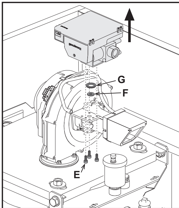
рис. 59 - Модель QUADRIFOGLIO B 70
