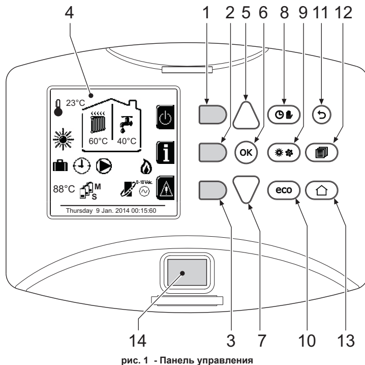
рис. 1 - Панель управления
