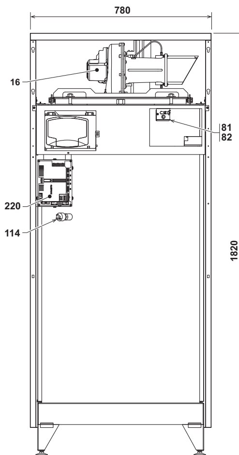
рис. 73 - Вид спереди модели B 220
