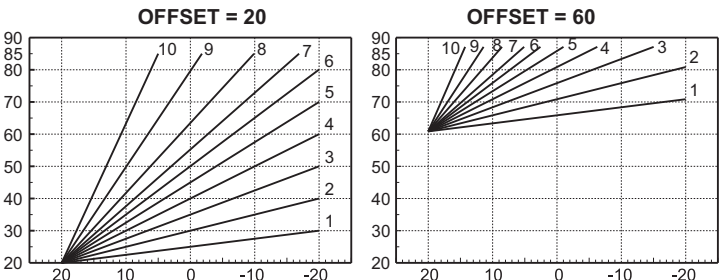
рис. 29 - Пример параллельного перемещения кривых погодозависимого регулирования
