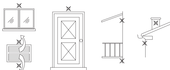
рис. 53 - Места, в которых не рекомендуется установить датчик температуры наружного воздуха.
