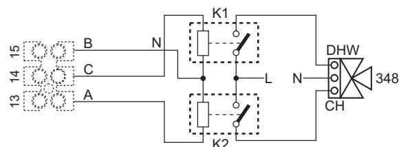
рис. 97- Подключение 3-х ходового клапана с 3 проводами
