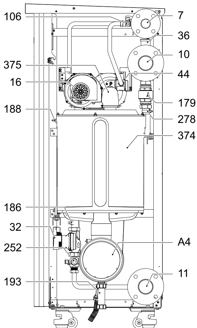
рис. 94- Основные компоненты
