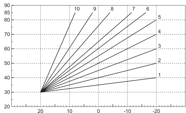
Рис. 1. Компенсационные кривые
