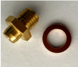
41560240-12 Переналадка на сжиженный газ d.0,82 mm
