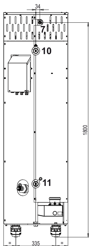
рис. 74- Вид сзади модели 70
