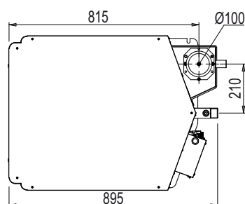
рис. 80- Вид сверху модели 125
