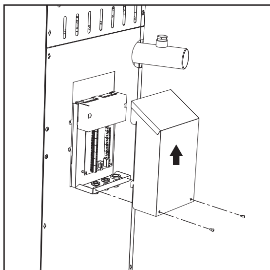
рис. 53- Клеммная колодка
