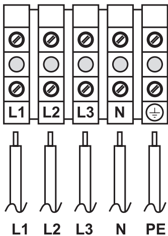
Рис. 21. Трехфазная проводка
