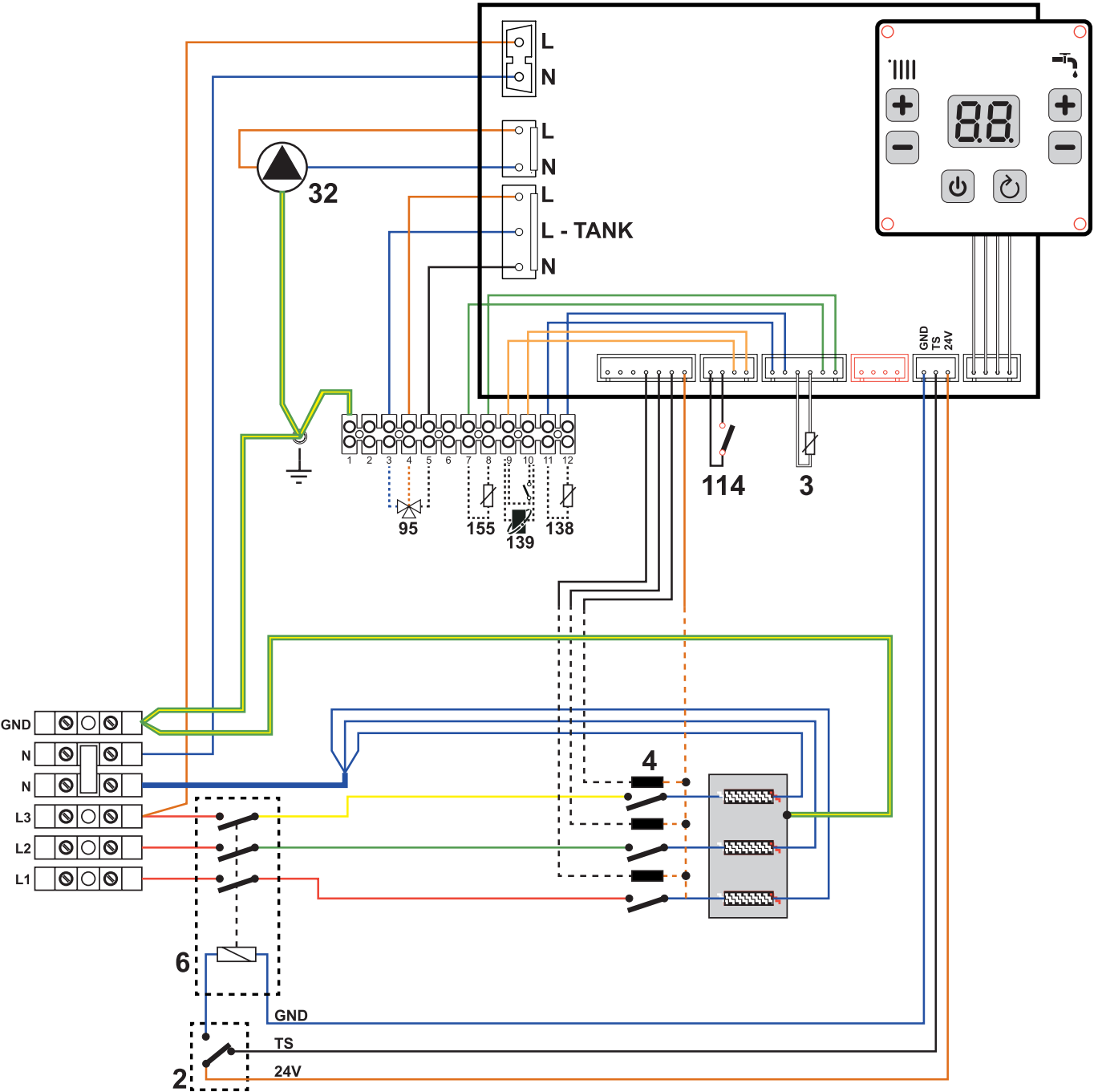
Рис. 19. Для моделей 6, 9 и 12 кВт 2) защитный термостат (ручной сброс); 3) датчик температуры отопления; 4) реле включения ТЭНов; 6) автомат защиты; 32) насос; 95) трехходовой кран (опция); 114) реле давления воды; 138) датчик уличной температуры (опция); 139) комнатный термостат / ПДУ с OpenTherm (опция); 155) датчик NTC бойлера (опция).
