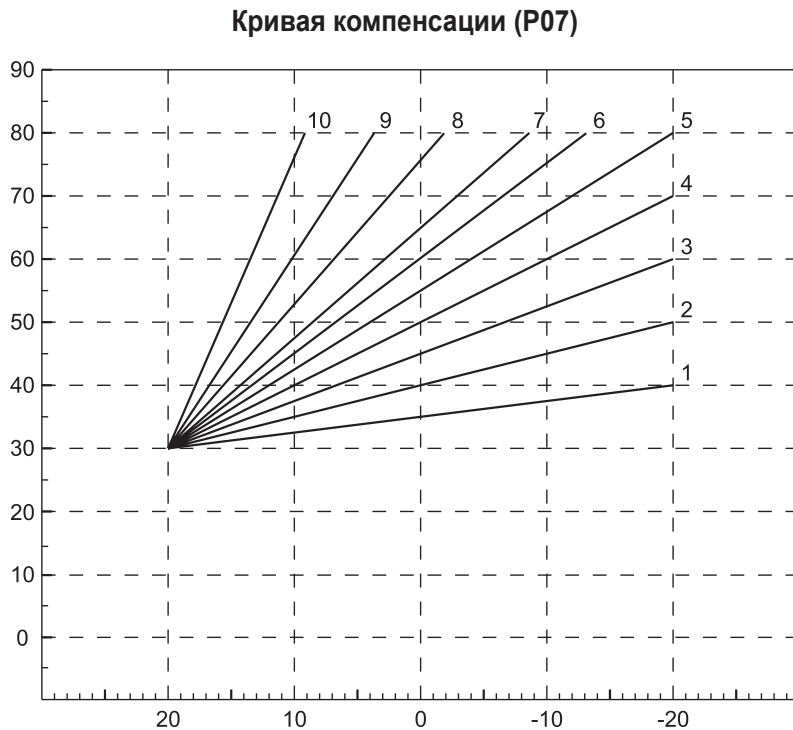
Рис. 2 Отопительные кривые. Смещение = 30 (установка по умолчанию).
