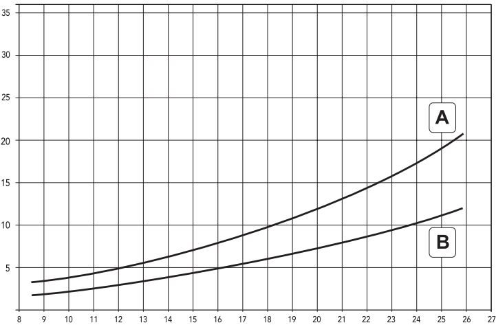
Рис. 17. Кривая давление газа/мощность A – сжиженный газ; B – метан
