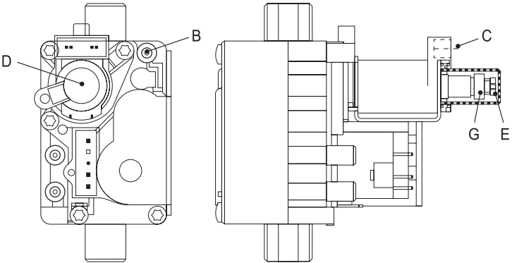
Рис. 13. Газовый клапан
