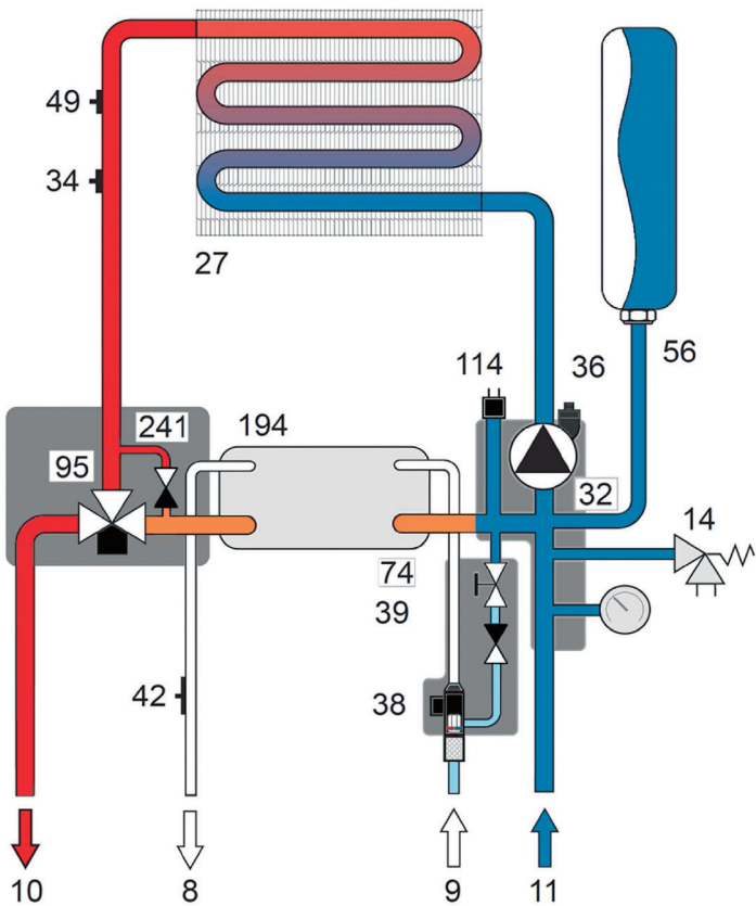
Рис. 15 Гидравлический контур
