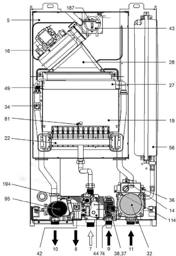
Рис. 14 Конструкция котла
