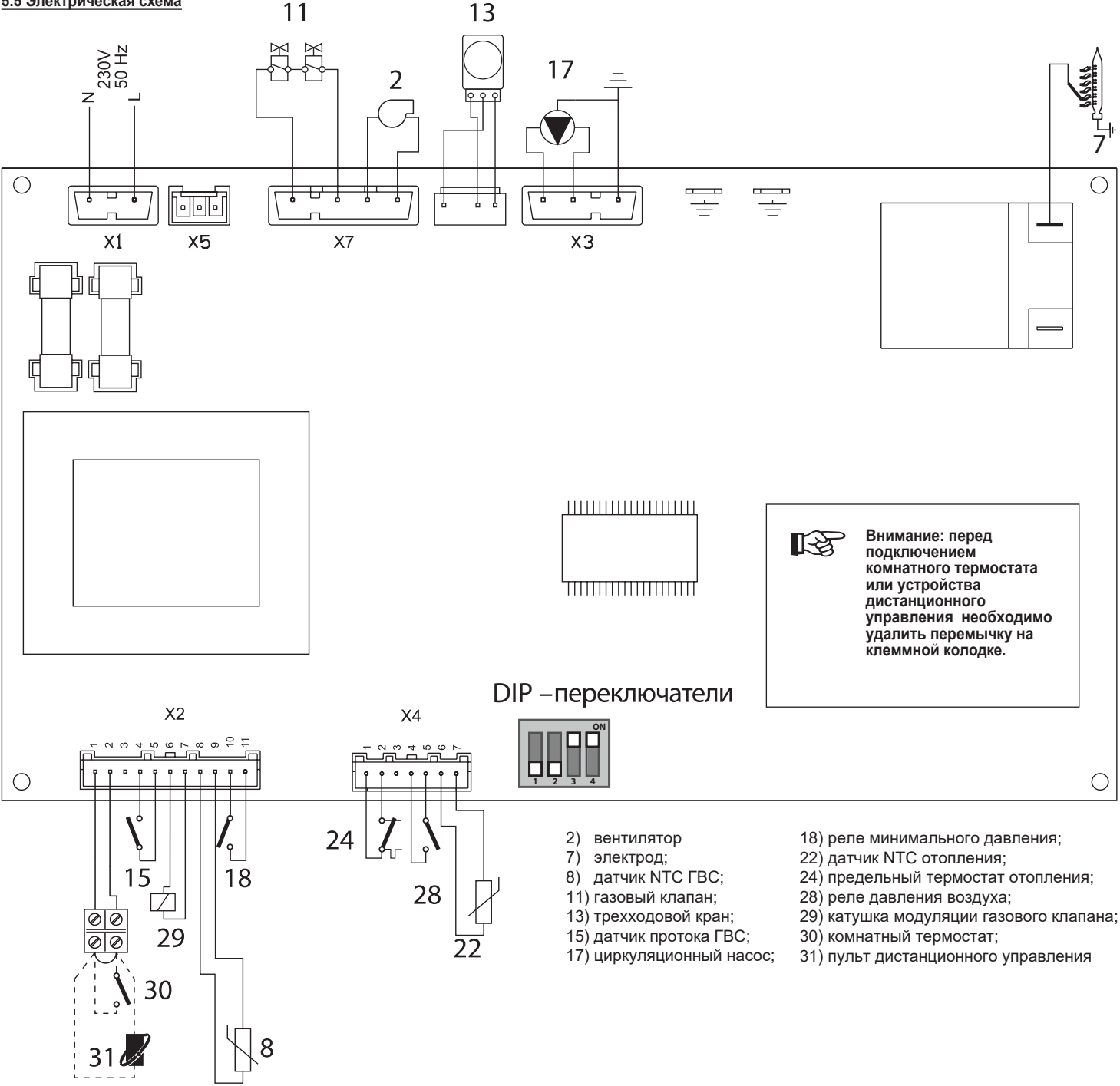
Рис. 20. Электрическая схема
