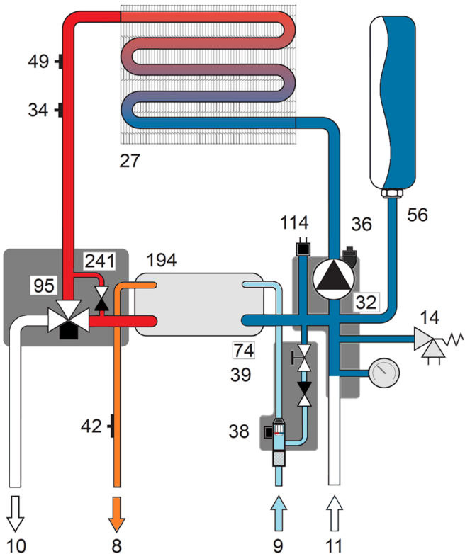
Рис. 19. Контур ГВС
