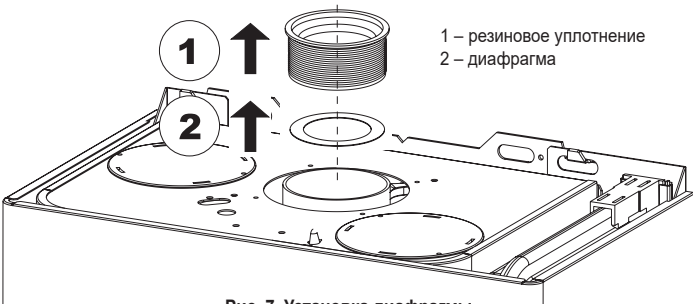
Рис. 7. Установка диафрагмы
