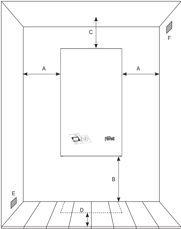
Рис. 5. Место установки
