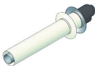
1 м труба горизонтальная оконечная с оголовком и защитной накладкой Ø100/150 мм 041110X0
