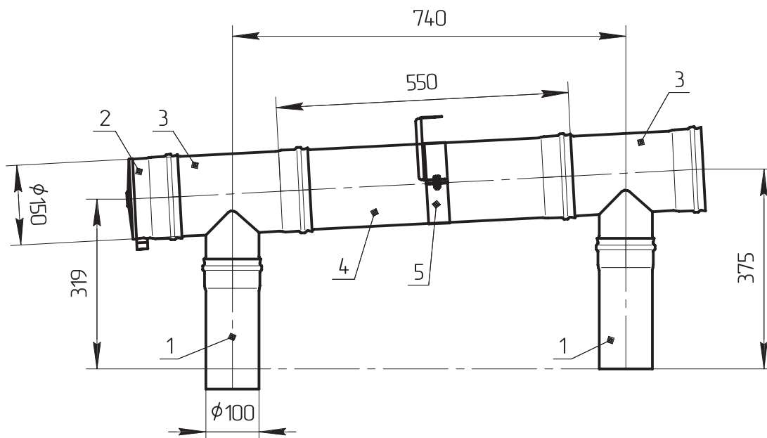
Спецификация для дымохода Ø150 мм (артикул 20211)
