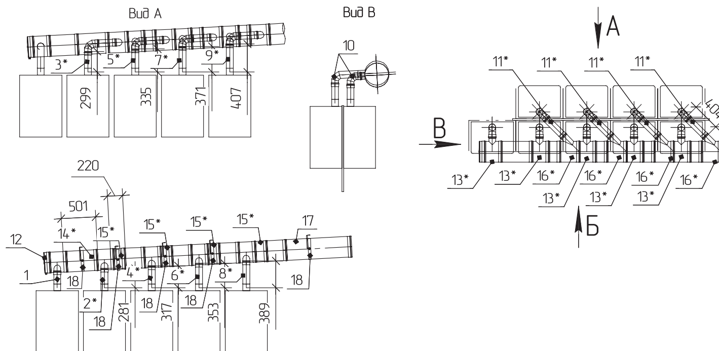
Спецификация для дымохода Ø300 мм
