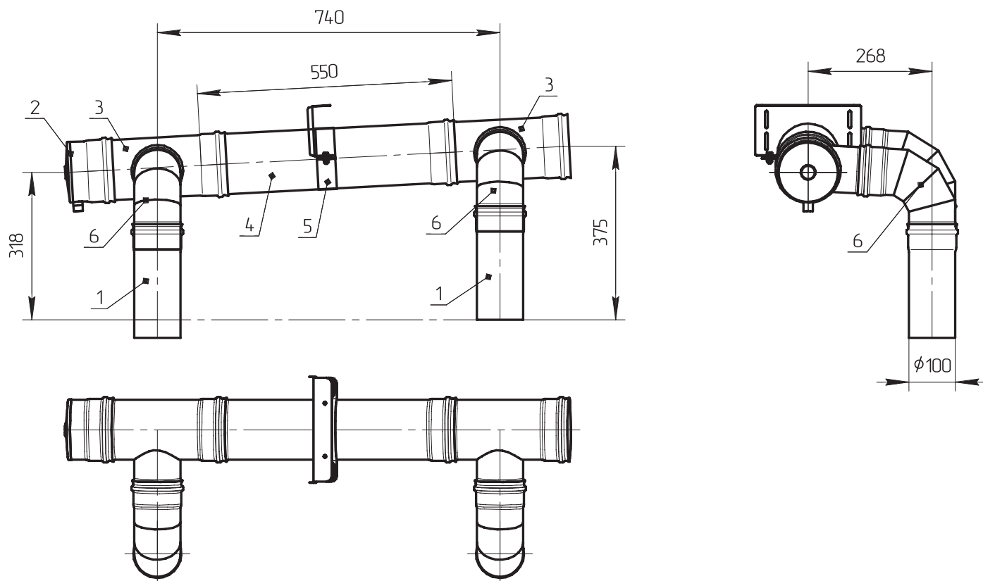
Спецификация для дымохода Ø130 мм (артикул 20112)
