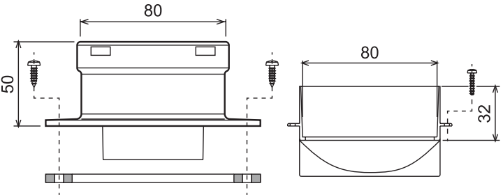
Рис. 11. Соединительный элемент для раздельного дымоудаления (арт. 01000)
