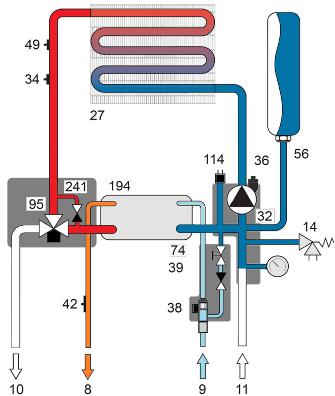
Рис. 19. Контур ГВС
