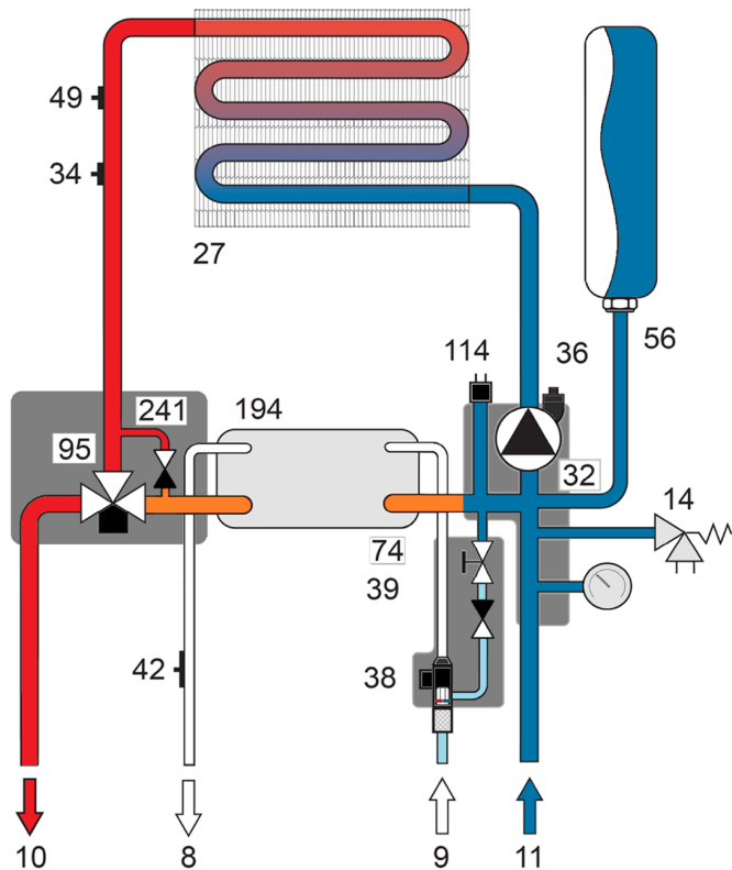
Рис. 18. Отопительный контур
