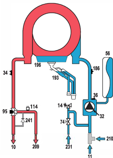
Рис. 41. Гидравлическая схема
