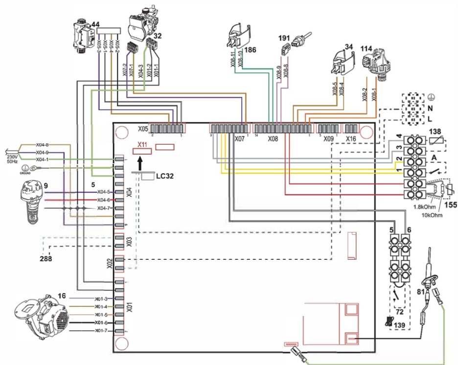
Рис. 45. Электрическая схема
