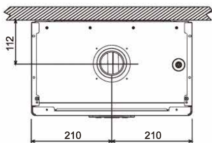
Рис. 34. Вид сверху
