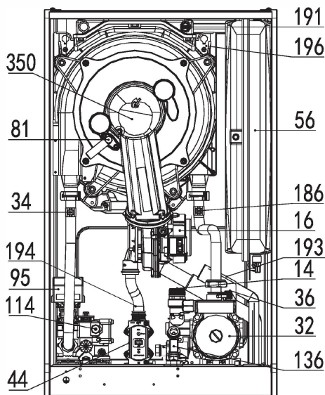
Рис. 40. Конструкция
