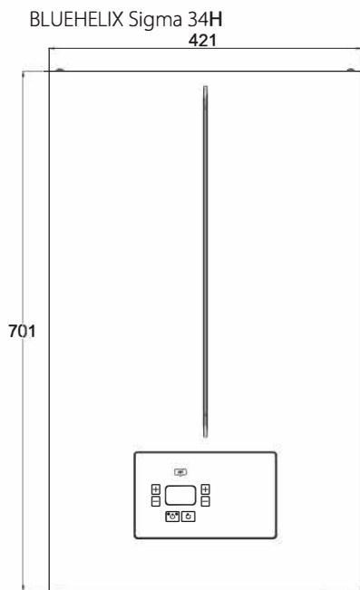
Рис. 36. Вид спереди
