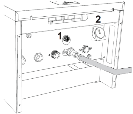
Рис. 16. Заполнение и подпитка системы отопления
