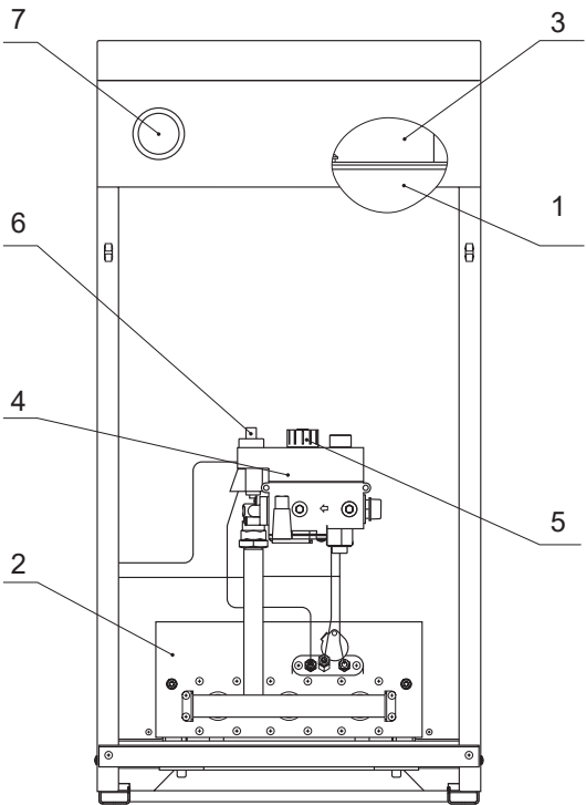
Рис. 2. Особенности котла с газовым блоком TGV 370 Модели котлов TORINO CLASSIC 10; 12,5; 16; 20
